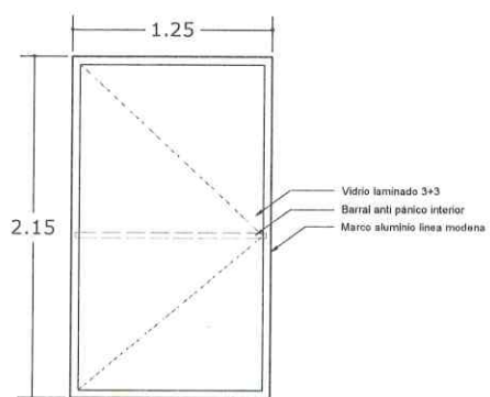
PUERTA DE ACCESO ESCUELA INFANTIL CANT: 1 UNIDAD
