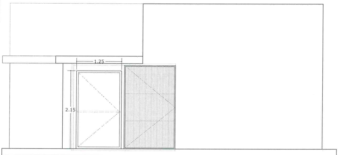
PUERTA DE ACCESO ESCUELA INFANTIL CANT: 1 UNIDAD
