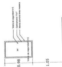
VIDRIO TIPO 4 CANT: 1 UNIDAD
