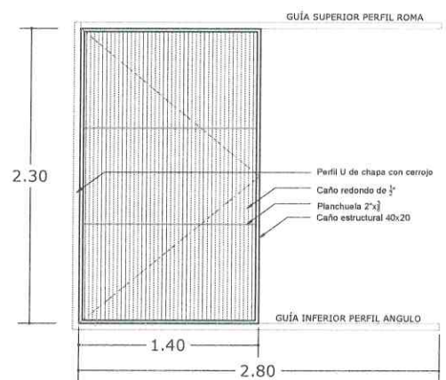
REJA DE ACCESO ESCUELA INFANTIL CANT: 1 UNIDAD
