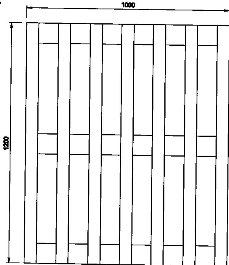
VISTA SUPERIOR
