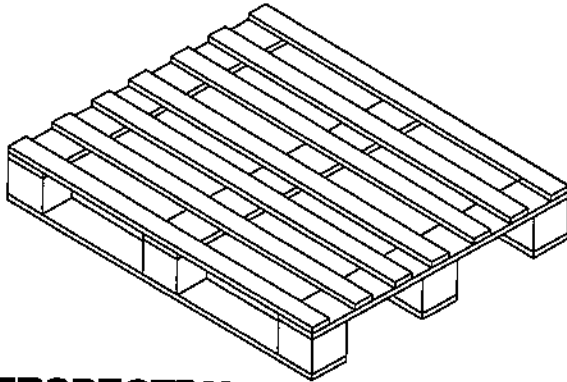
PERSPECTIVA
