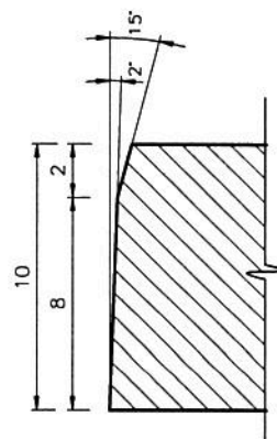
DETALE " " Scala 5:1
