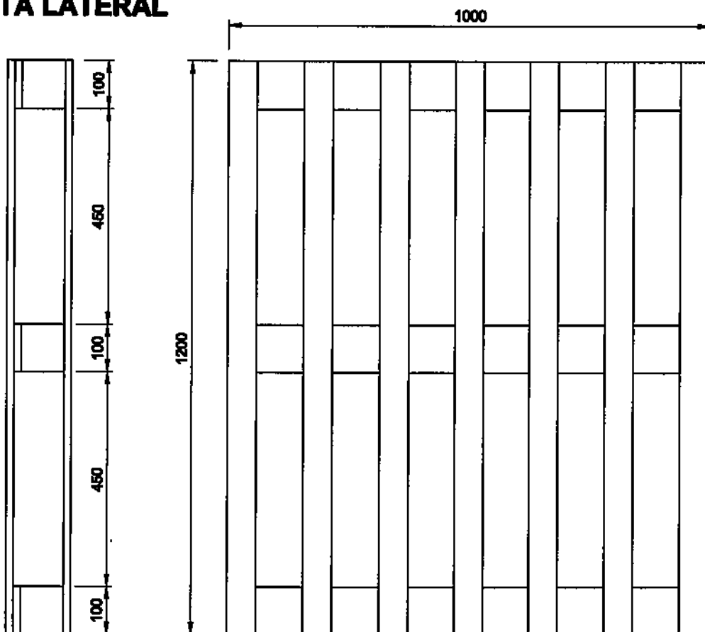
VISTA SUPERIOR
