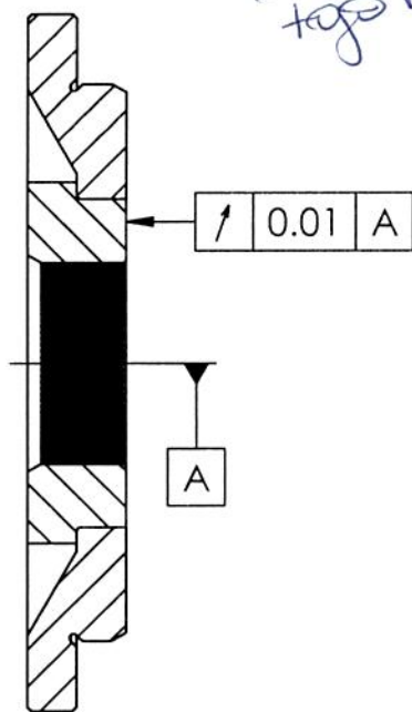
SECCIÓN A-A
