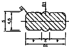
CORTE, escala 4:1
