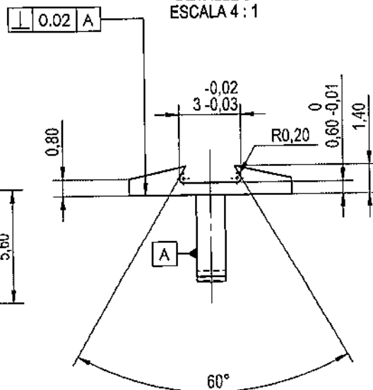
DETALLE B ESCALA 4:1
