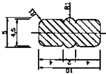
CORTE, escala 4:1
