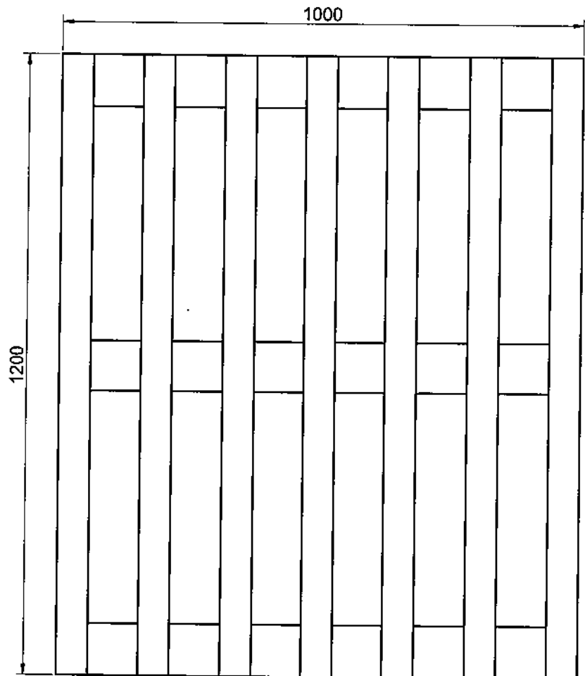
VISTA SUPERIOR
