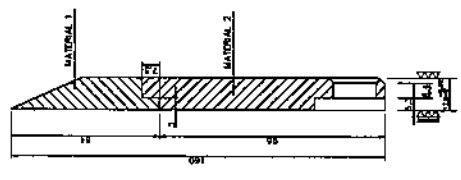
CORTE A-A Escala 1:1
