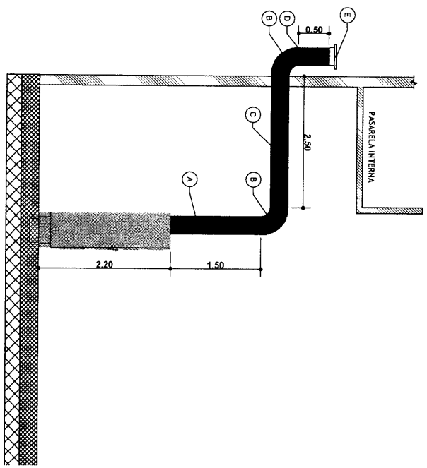
CORTE A-A LÍNEA DE CONDUCTOS Ø300 mm
