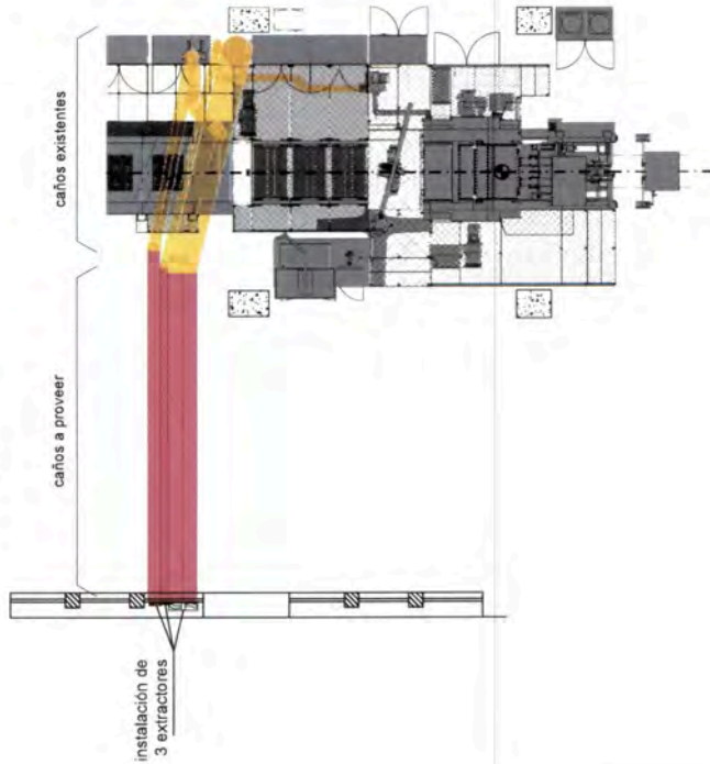
VISTA PLANTA
