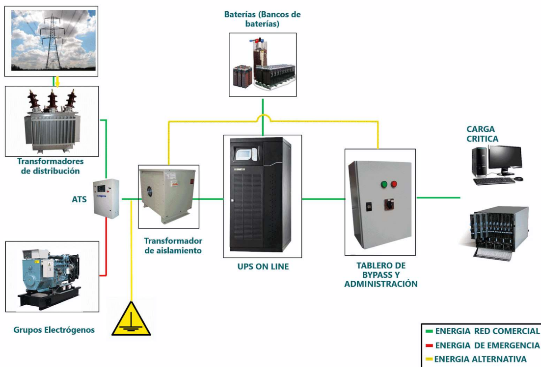
ESQUEMA DE PROTECCION ELECTRICA PARA SU CARGA CRITICA
